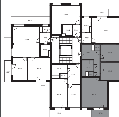
UMÍSTĚNÍ BYTU NA PODLAŽÍ
